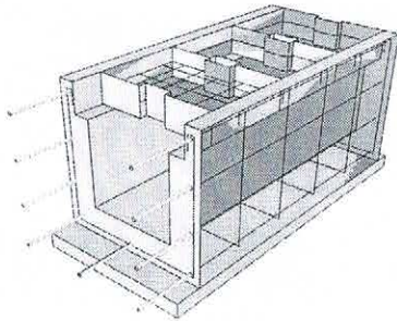
แบบทัศนียภาพรางระบายน้ำ
