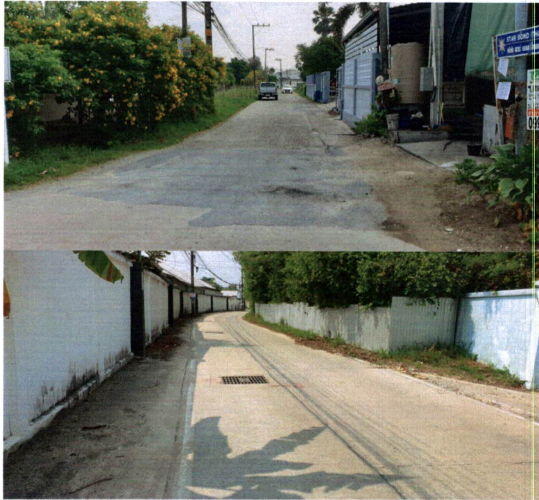
รูปก่อนดำเนินงานโครงการก่อสร้างถนนแอสฟัลท์ติกคอนกรีต บริเวณซอยโรงกาว ม.๕ ต.นาป่า
