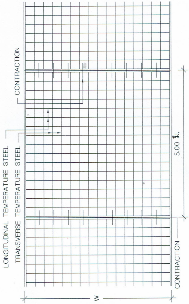
แปลนแสดงการเสริมเหล็กลาน ดสล. SCALE 1:75
